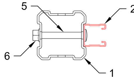
03 SECTION N.T.S.
